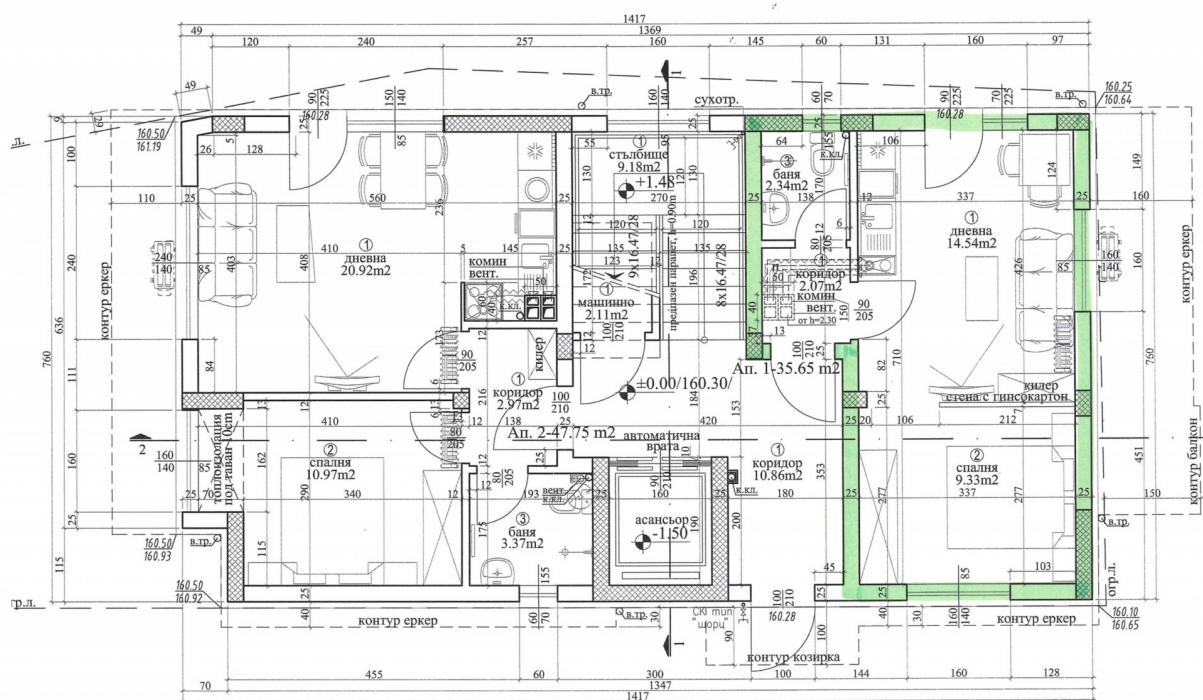
План на 1 етаж (к.±0.00/160.30/) З.П.=111.25 м2
