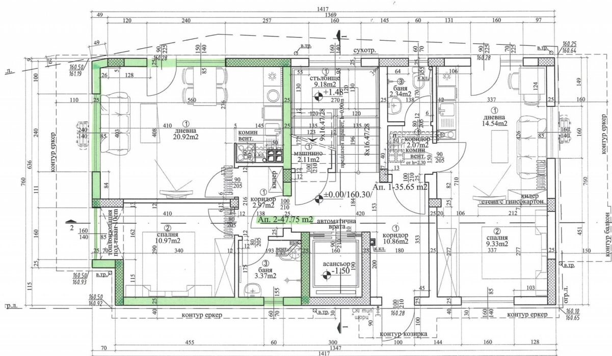
План на 1 етаж (к.±0.00/160.30/) З.П.=111.25 м2
